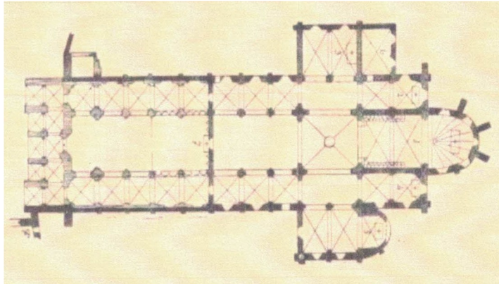
Plan de l'église abbatiale, fin XIème siècle, P. de Farcy, 1886, p. 40
